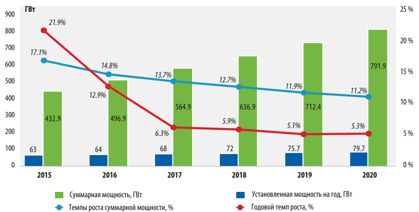
Рис. 3. Прогноз развития рынка мировой ветроэнергетики на 2016–2020 годы; (Источник: GWEC/2016)
